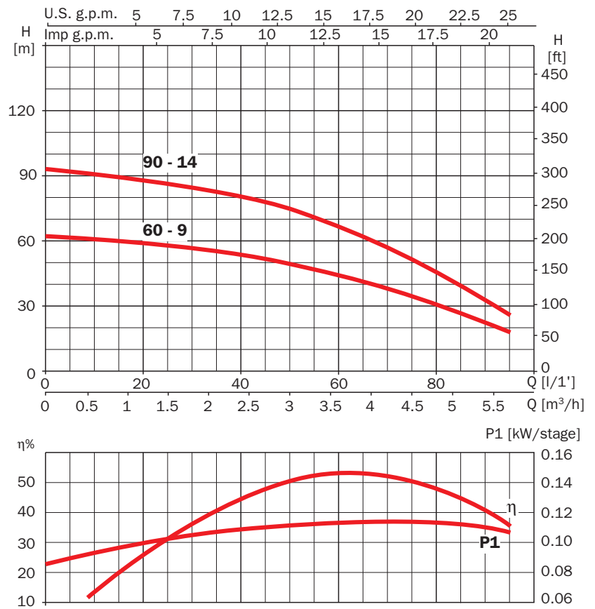
Curvas de funcionamiento a 2900 r.p.m. Performance curves at 2900 r.p.m.
