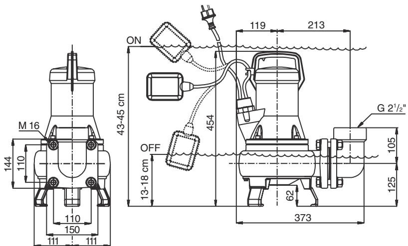
DRAINEX 300
