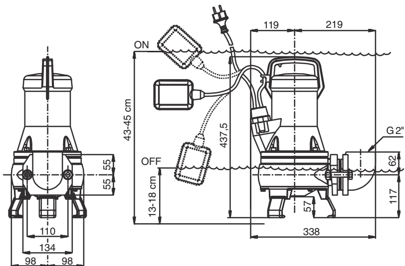
DRAINEX 200 / DRAINCOR
